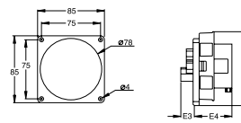
Ölçüler (mm)
