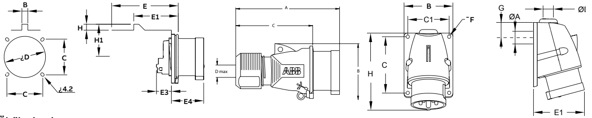
Ölçüler (mm)
