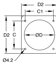
Ölçüler (mm)
