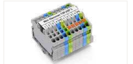
Geçmeli montaj ayaklı klemensleri
